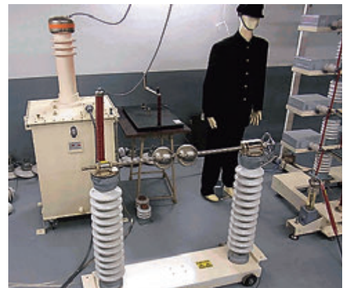
高電圧絶縁破壊実験
