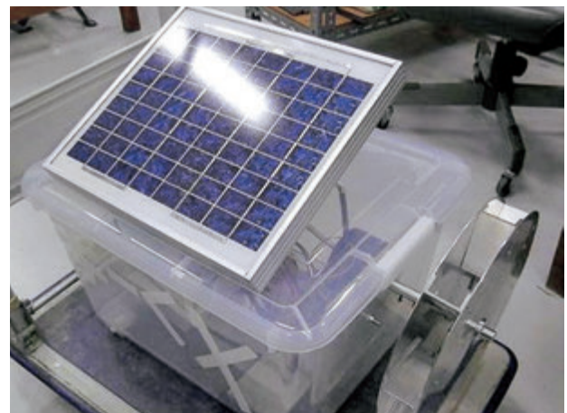
蓄電池を備えた太陽光・水力ハイブリッド発電機 （創造工学特別実験の試作品）
